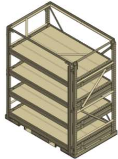
Glide-Out Module 3
