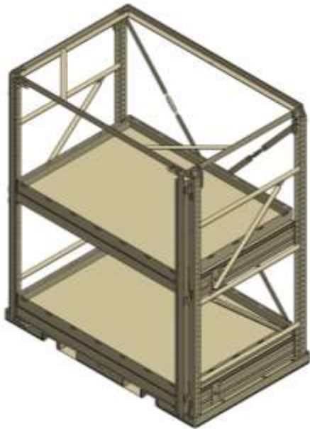
Glide-Out Module 4
